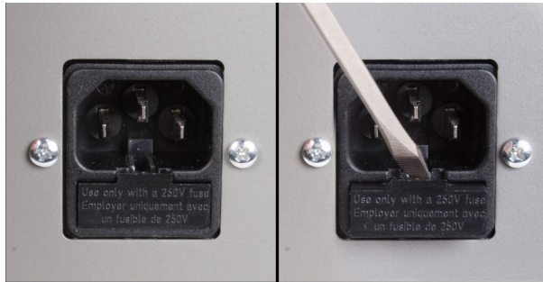
Módulo de entrada de energía Extracción de portador de fusibles
